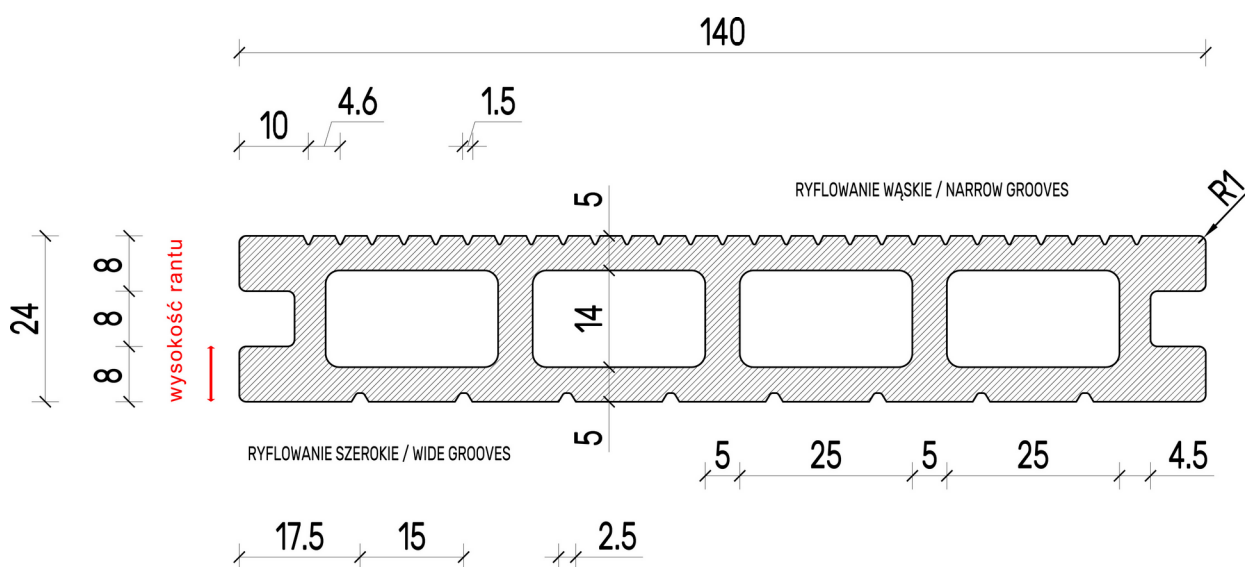
Rysunek A1. Deska tarasowa
